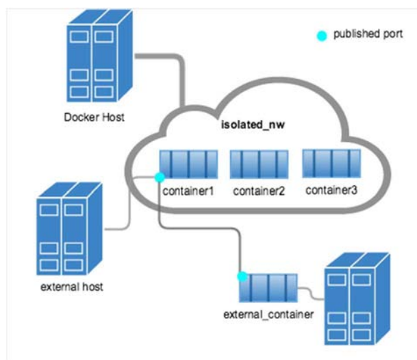
Figure 12 : schéma de publication des ports
