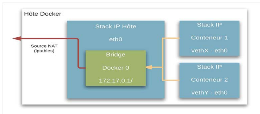
Figure 10 : Réseaux Bridge
