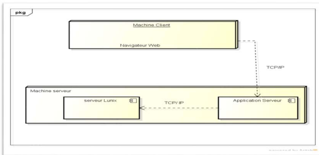
Figure 18 : Diagramme de déploiement
