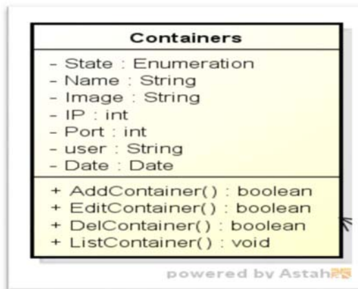
Figure 20 : classe contenaires
