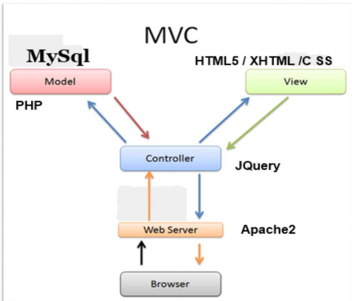
Figure 30 : Modèle MVC
