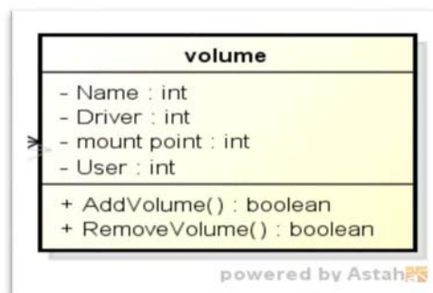
Figure 23 : Classe Volume
