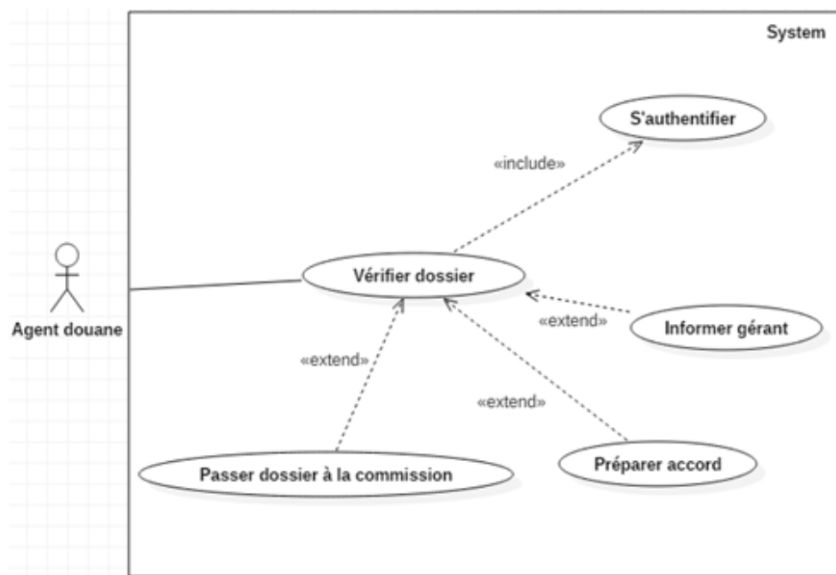
Figure 5: Diagramme de cas d'utilisation vérifier dossier
