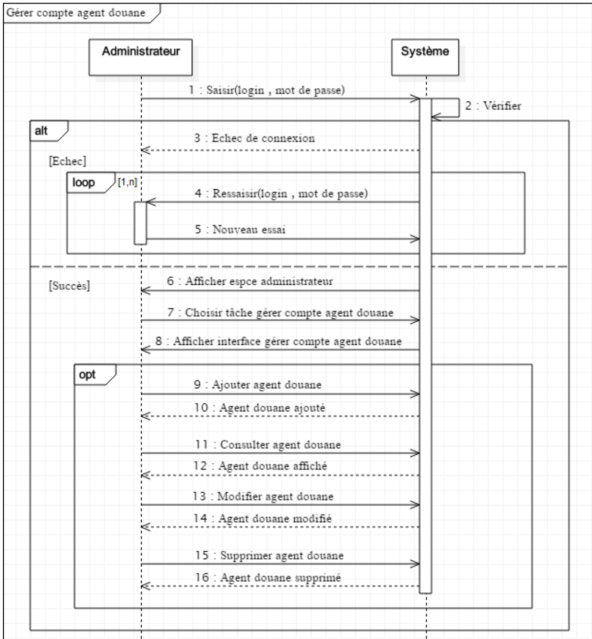
Figure 6: Diagramme de séquence du cas gérer compte agent douane
