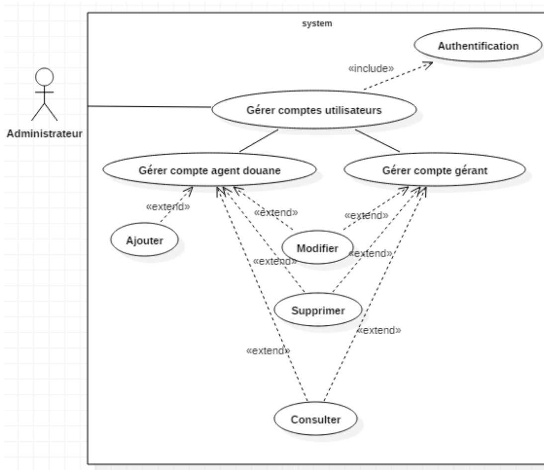
Figure 4: Diagramme de cas d'utilisation gérer comptes utilisateurs
