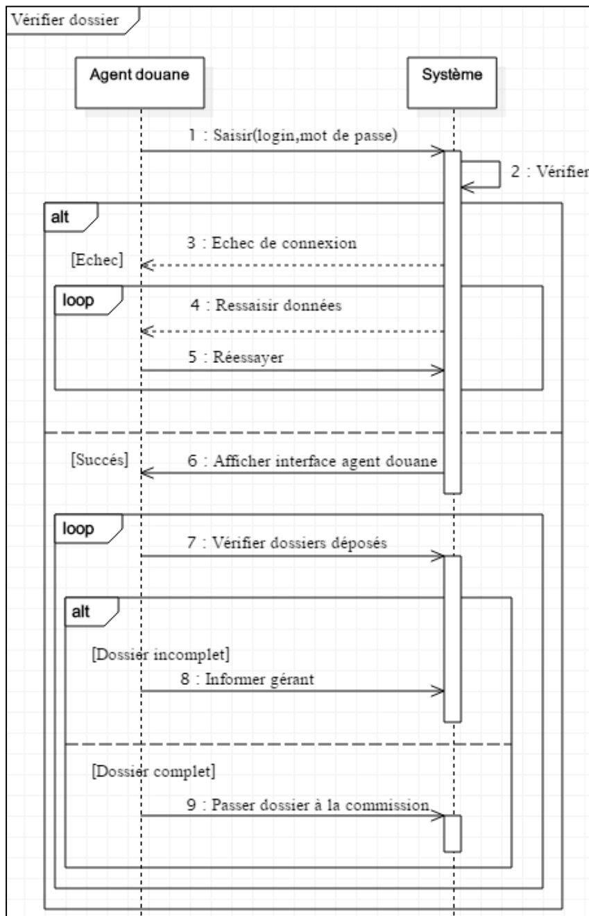
Figure 10: Diagramme de séquence du cas vérifier dossier
