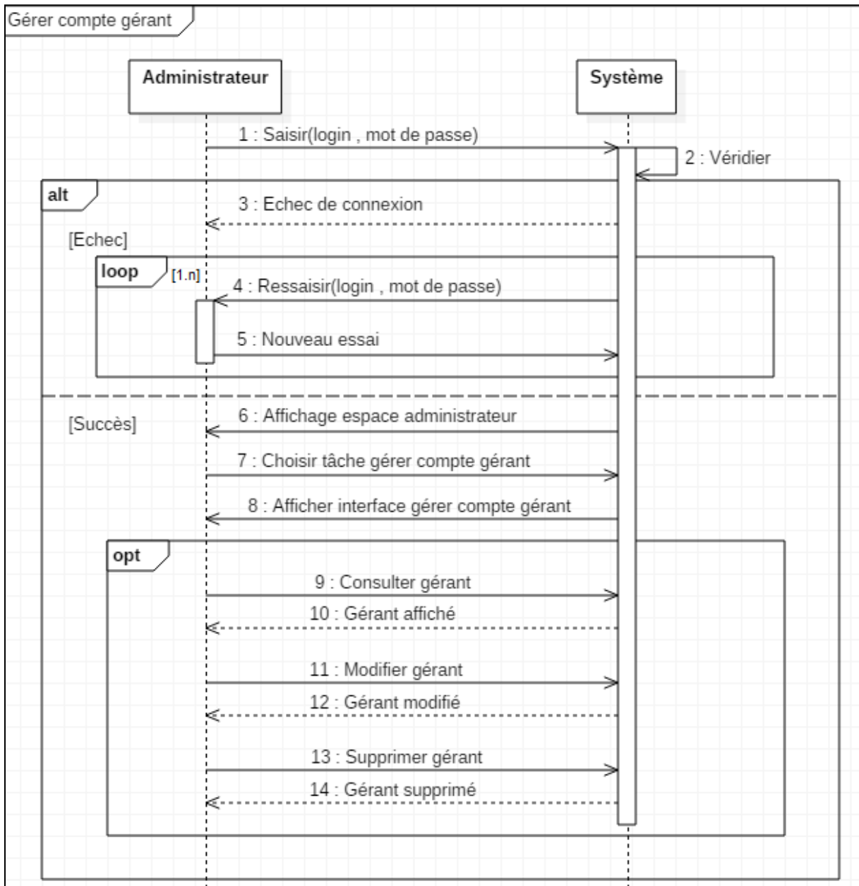
Figure 7: Diagramme de séquence du cas gérer compte gérant
