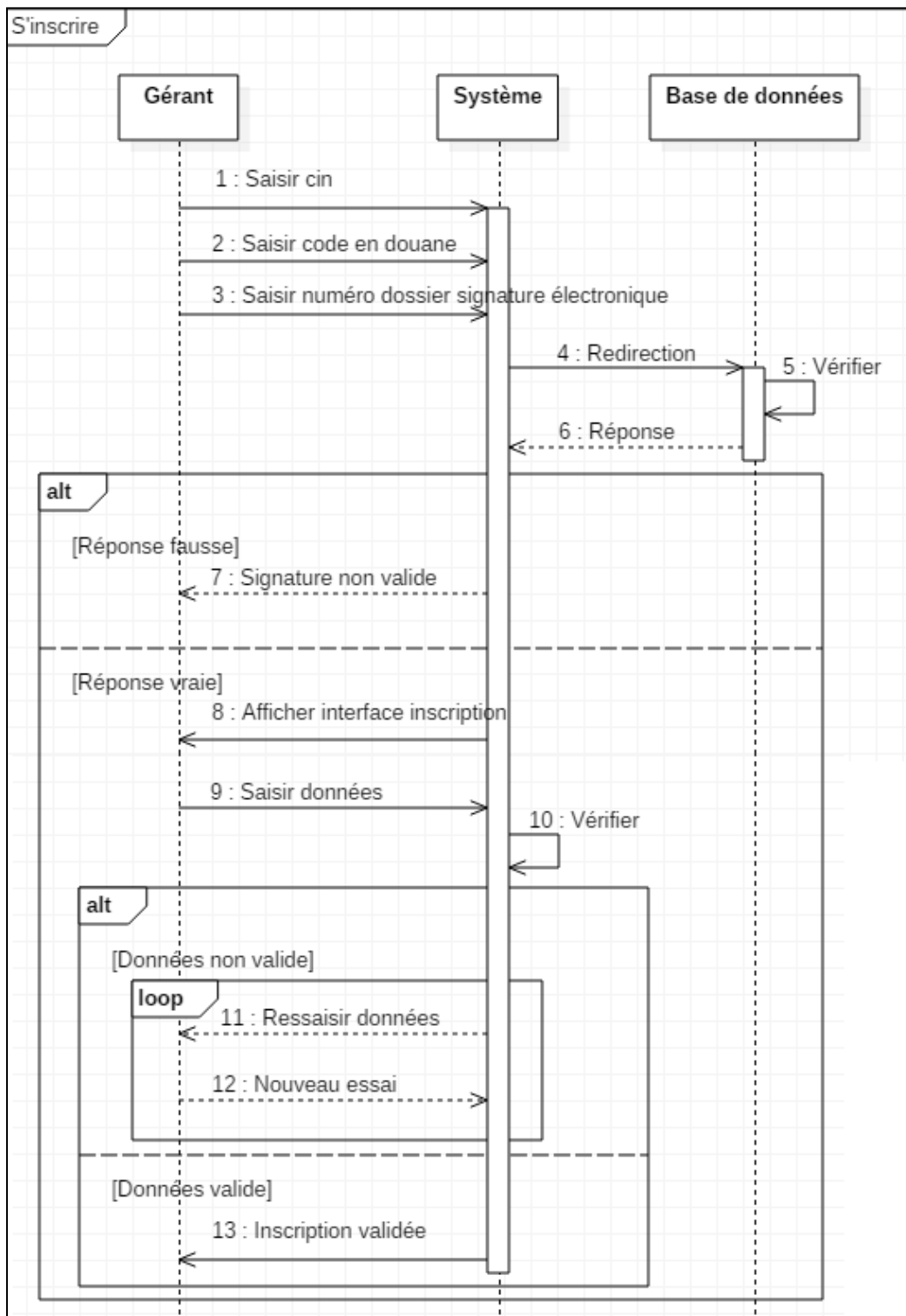
Figure 8: Diagramme de séquence du cas s'inscrire
