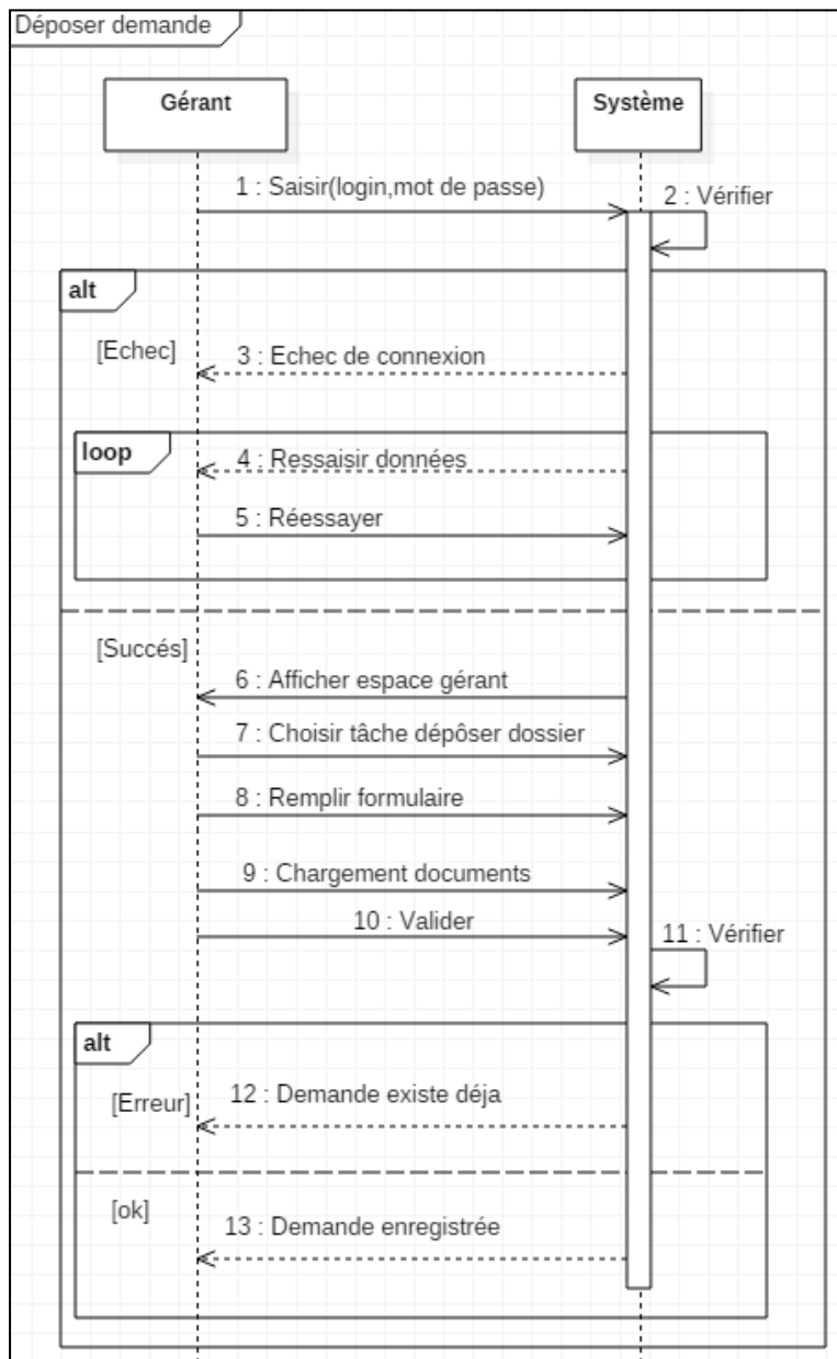
Figure 9: Diagramme de séquence du cas déposer une demande
