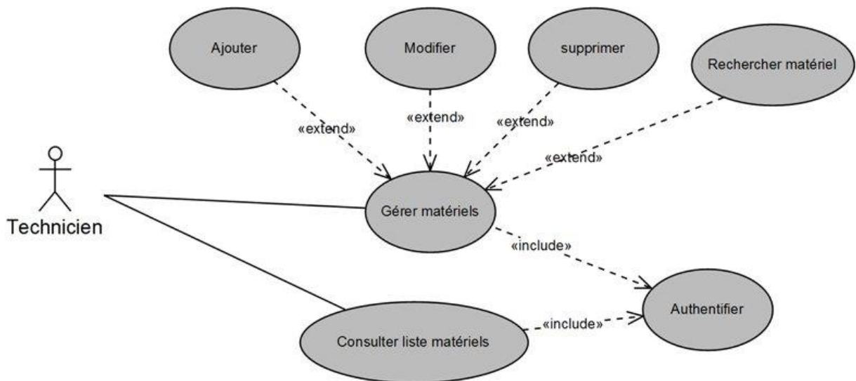
Figure 5: Diagramme de cas d'utilisation : Gérer matériels
