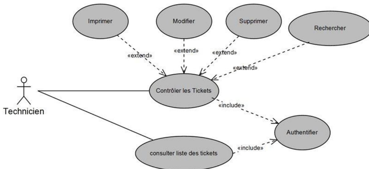
Figure 9: Diagramme de cas d'utilisation : Contrôler les Tickets
