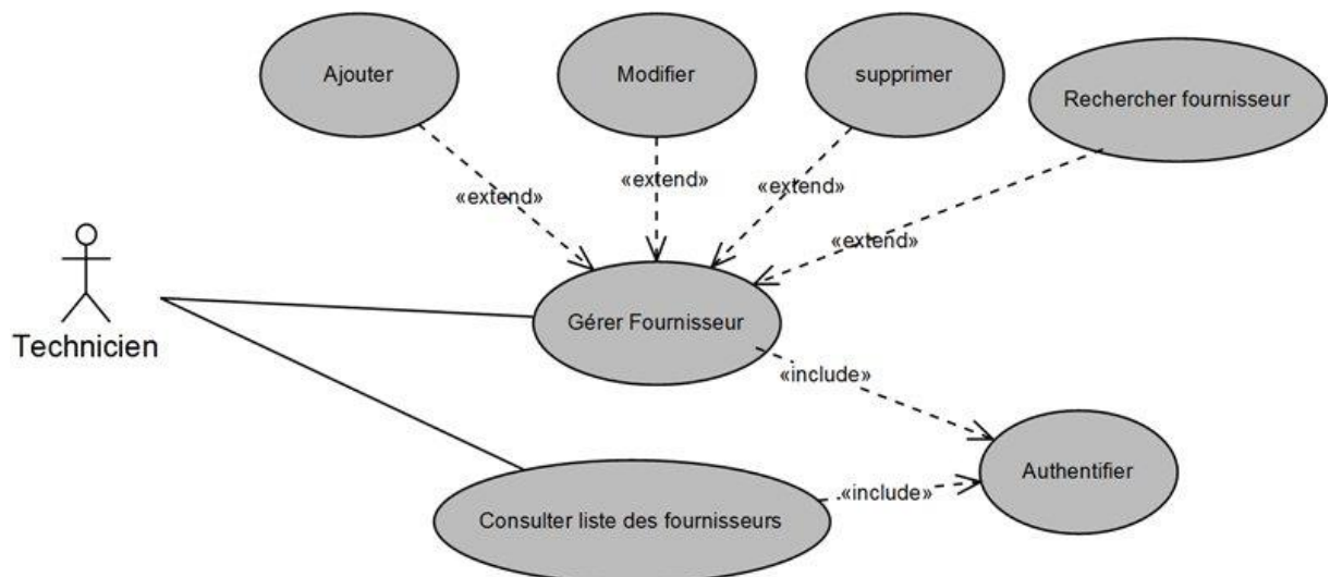
Figure 7: Diagramme de cas d'utilisation : Gérer Fournisseur
