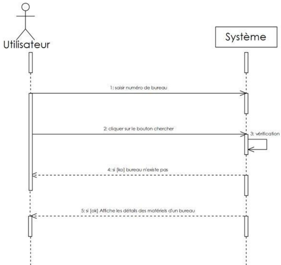
Figure 13: Diagramme de séquence pour le cas d'utilisation « consultation des matériels d'un bureau »
