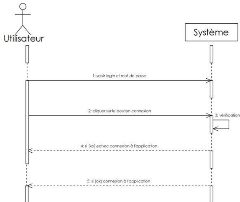
Figure 11: Diagramme de séquence pour le cas d'utilisation « authentification »
