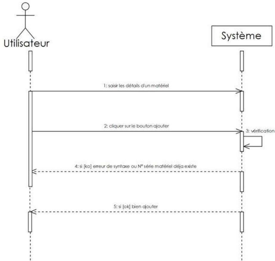
Figure 12: Diagramme de séquence pour le cas d'utilisation « ajout d'un nouveau matériel »
