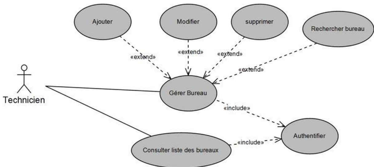
Figure 6: Diagramme de cas d'utilisation : Gérer Bureau
