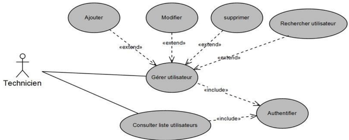
Figure 4: Diagramme de cas d'utilisation : Gérer utilisateurs
