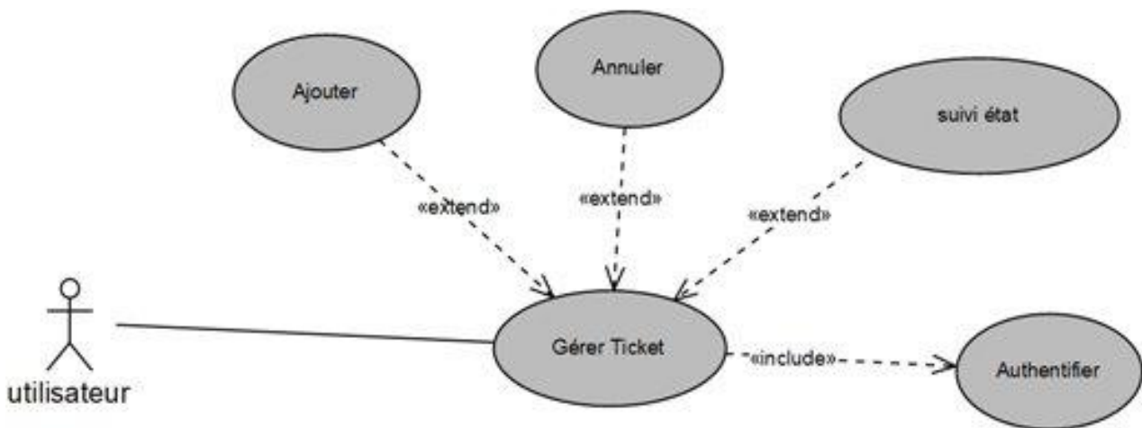
Figure 8: Diagramme de cas d'utilisation : Gérer Ticket par un utilisateur
