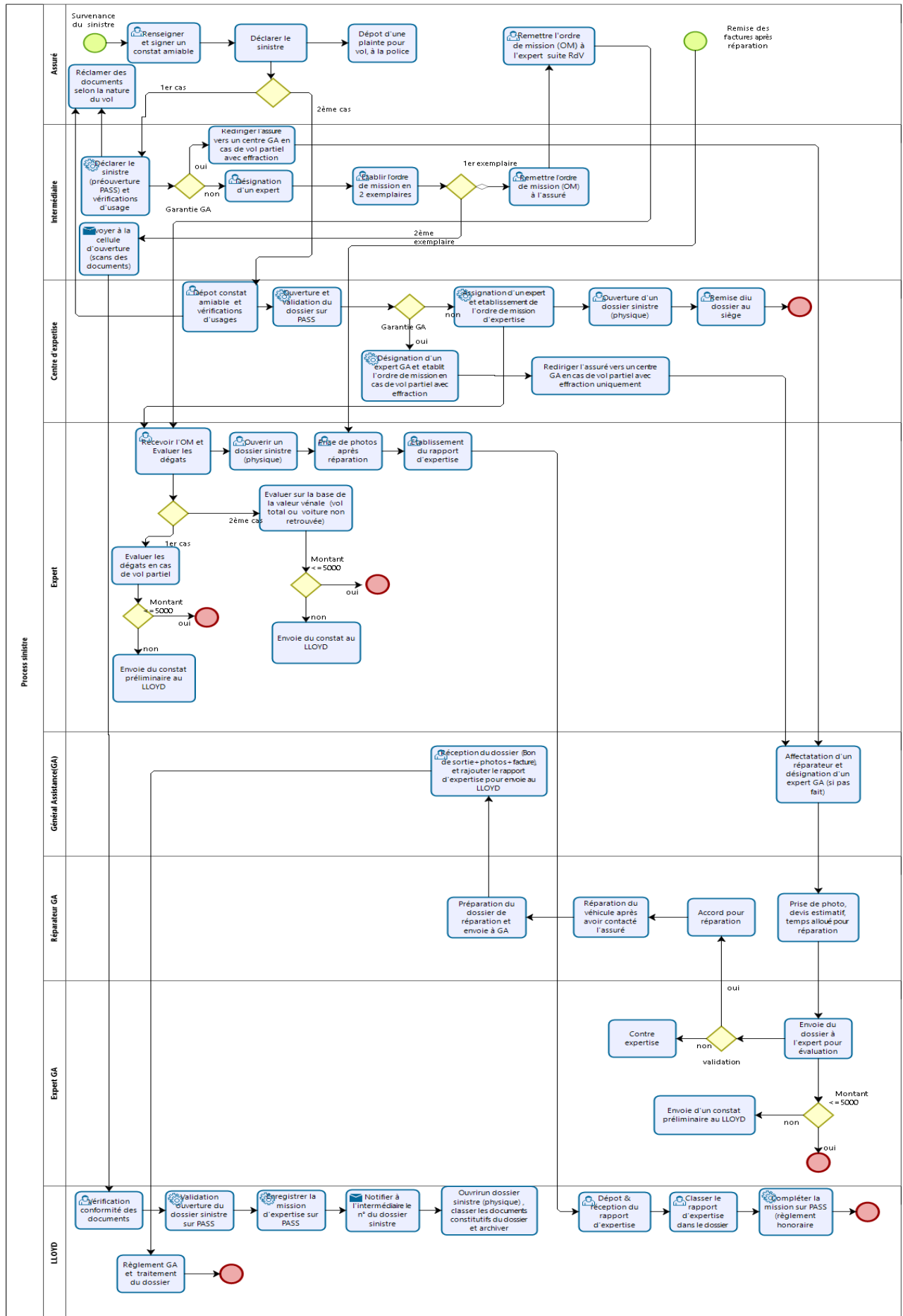
Figure 19. Processus Déclaration d'un sinistre vol automobile
