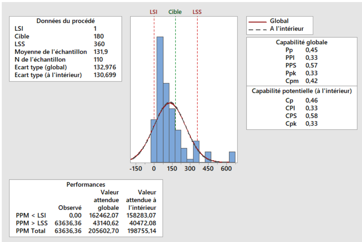
Figure 27. Capabilité du processus sinistre auto
