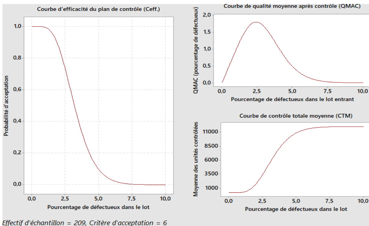
Figure 31. Plans de contr  le par attributs
