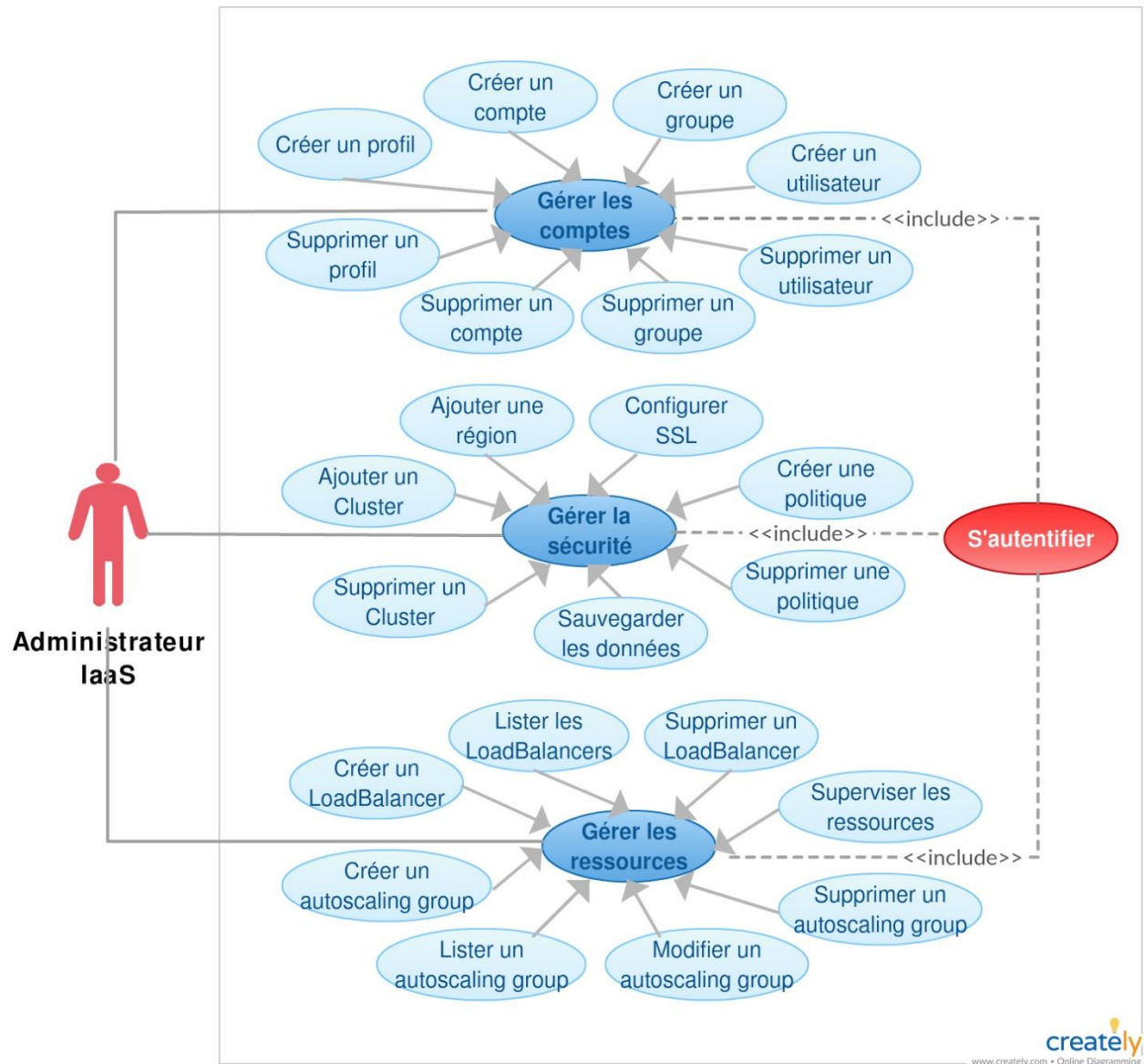
Figure 3.5: Diagramme de cas d'utilisation générale relatif à l'admin
