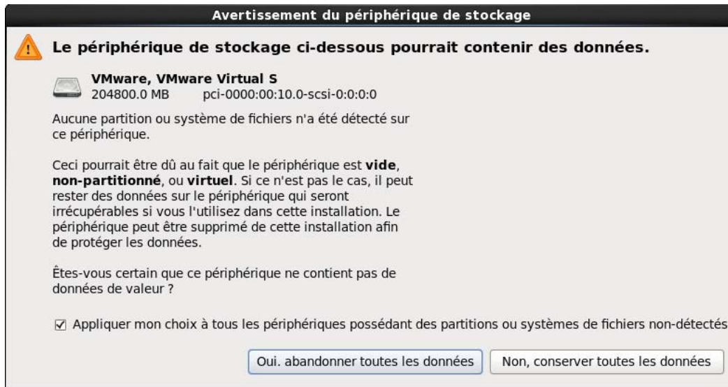
Figure 0.3-Formatage du disque
