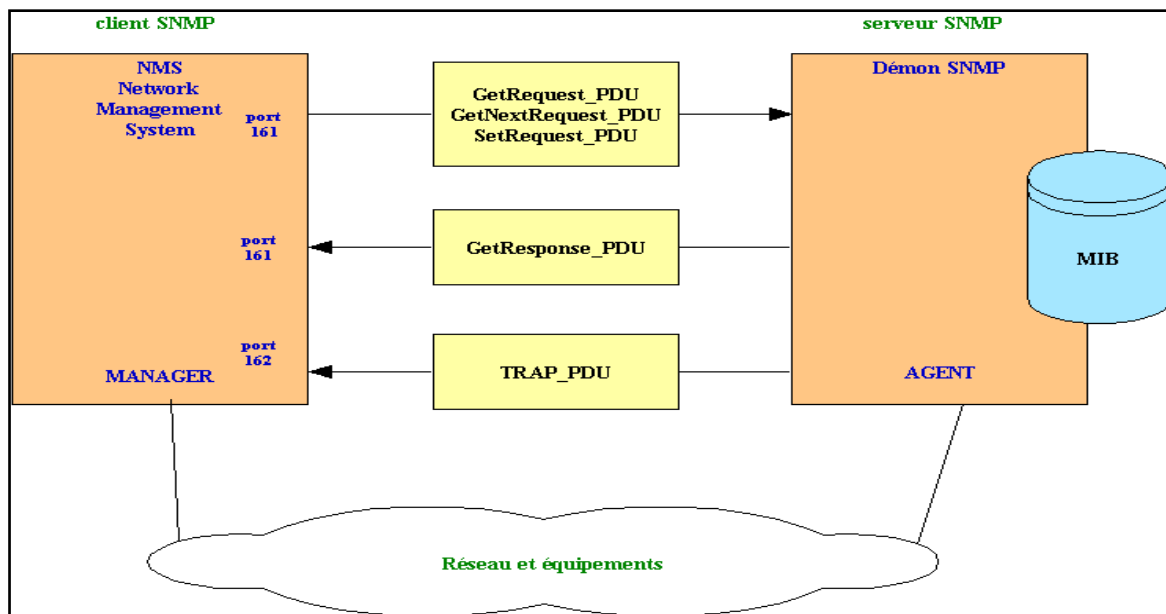
Figure 6 : fonctionnement SNMP
